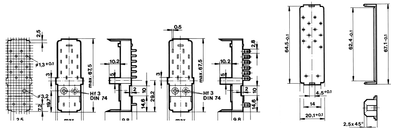
Demontagehilfe für H-462/2 Bestellnummer: 462 – 8006 Removal tool for H-462/2 Ordering number: 462 – 8006
