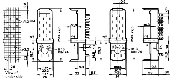
Fassung H-464/3 mit Lötflähen mit Lötstiften für Leiterplatten
